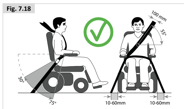
Fig. 7.18 Pour une utilisation exclusive avec le système d'arrimage Dahl (Fig. 7.18)
